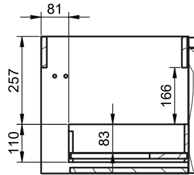
B-B ( 1 : 10 )
