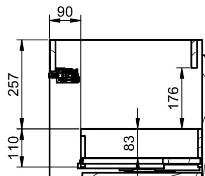
B-B ( 1 : 10 )
