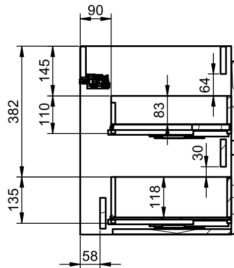
B-B ( 1 : 10 )
