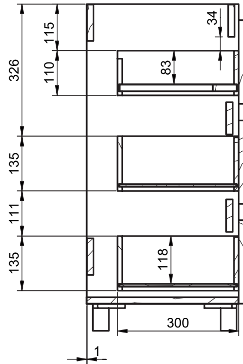
B-B (1 : 8)
